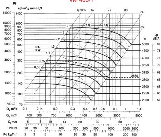
VM 400/T
