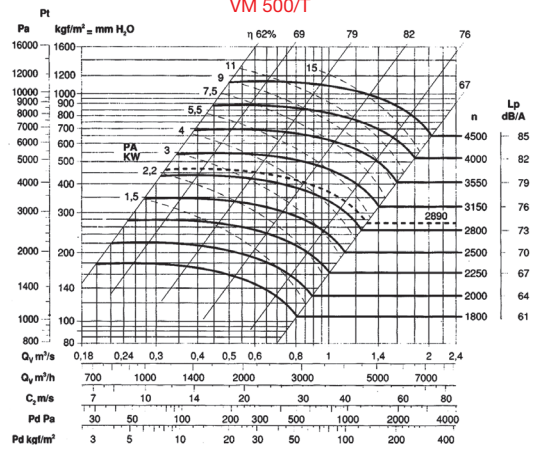
VM 500/T
