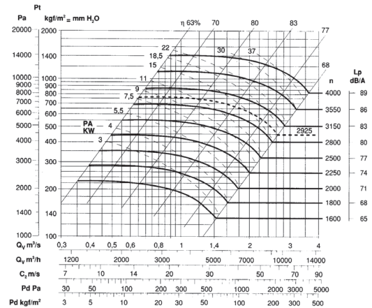
VM 630/T
