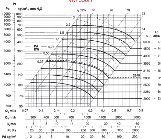
VM 350/T
