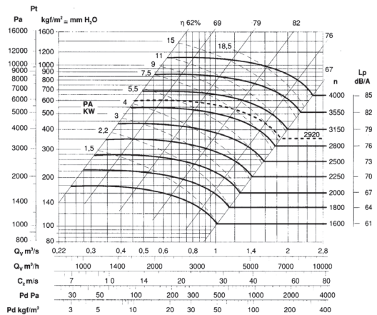
VM 560/T
